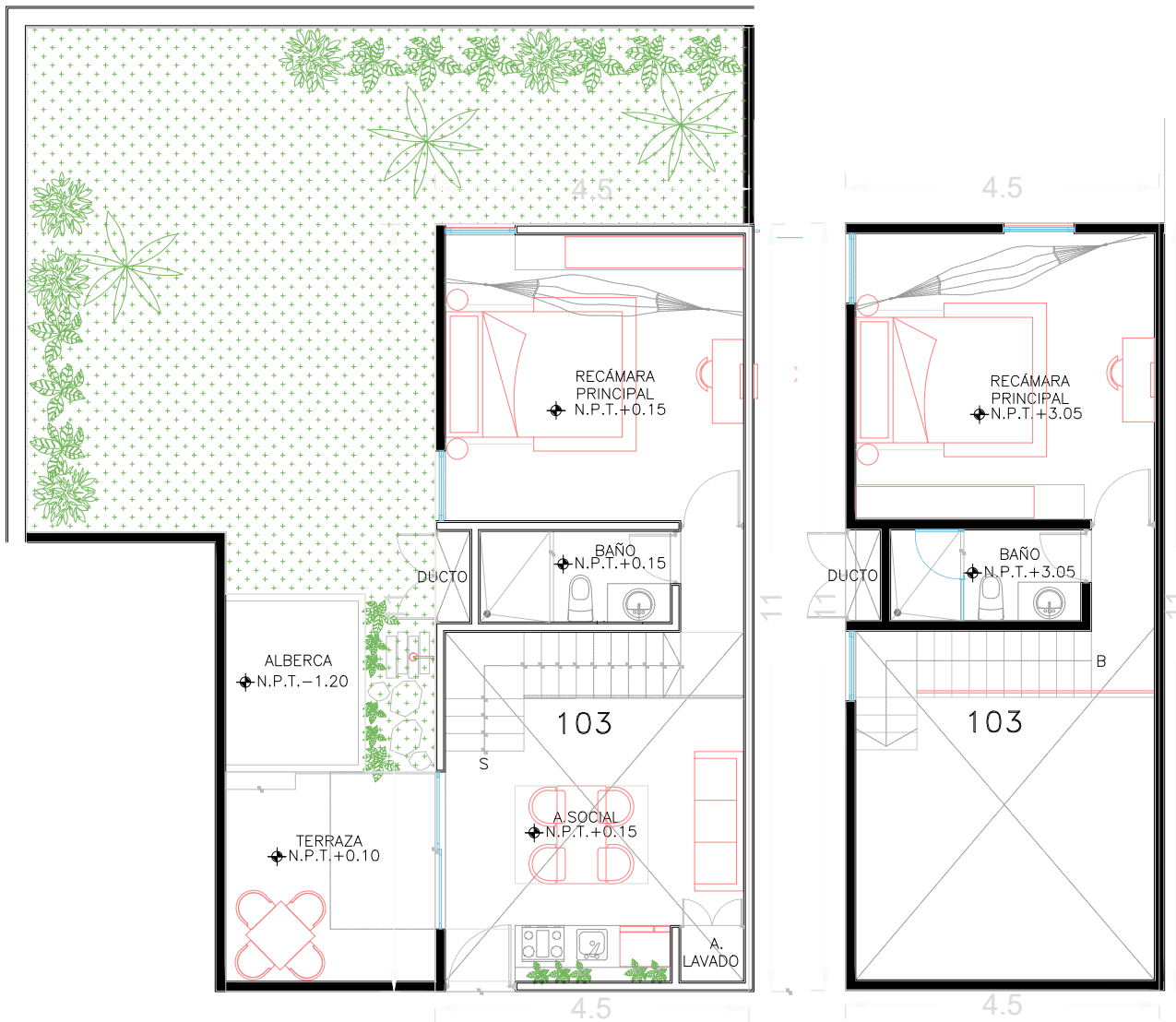
PLANTA BAJA
