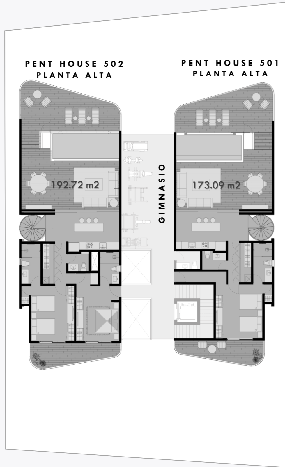
PLANTA ARQUITECTÓNICA ROOF GARDEN
