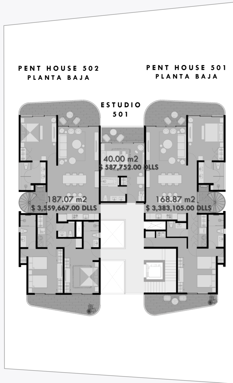
PLANTA ARQUITECTÓNICA NIVEL 5
