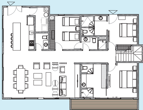
Planta Baja
