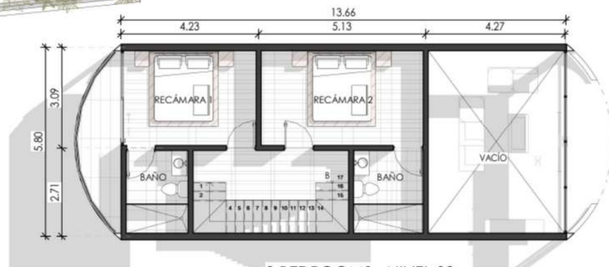
3 BEDROOMS - NIVEL 02
