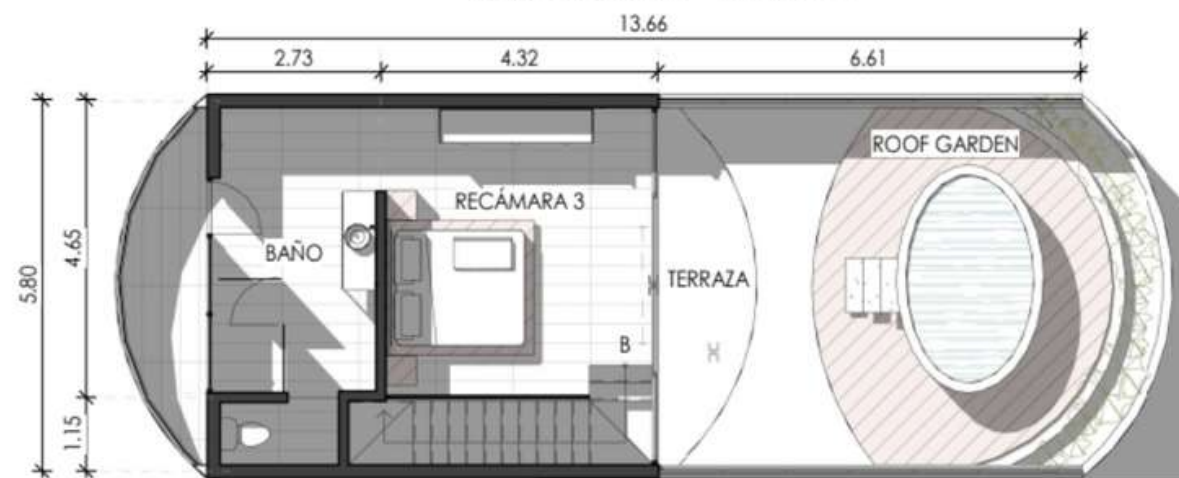
3 BEDROOMS - NIVEL 03
