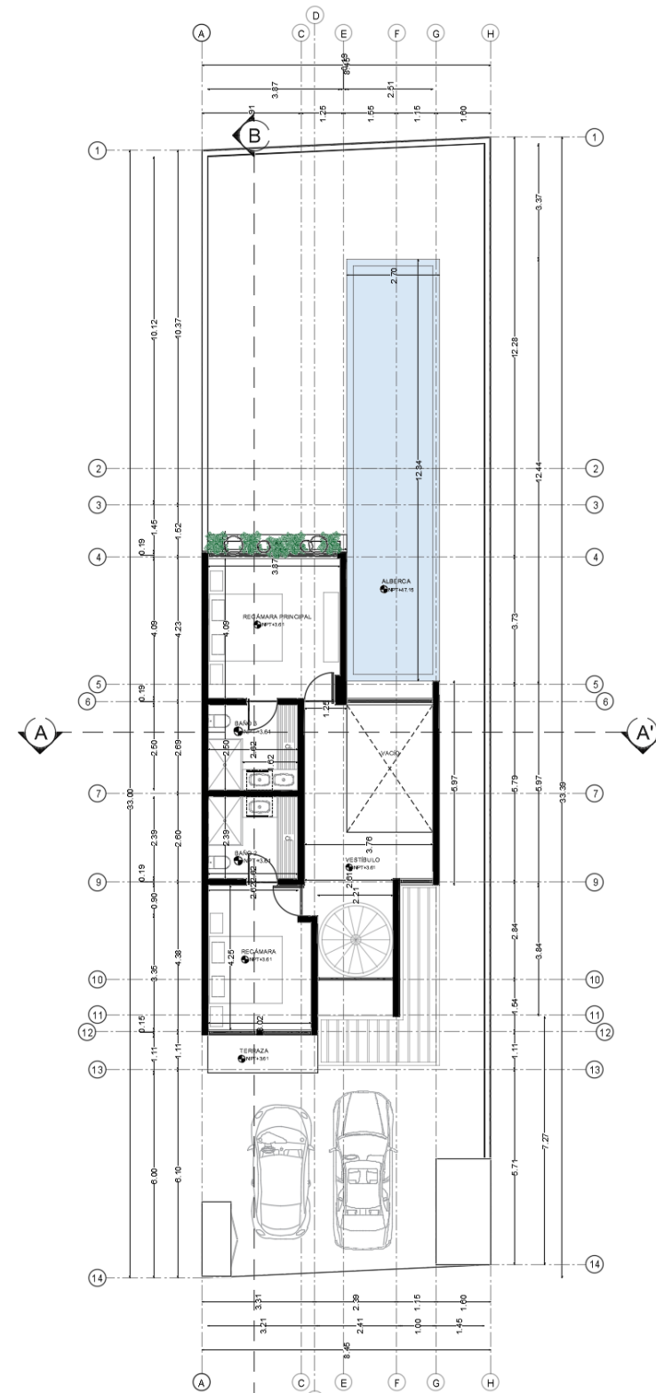
PLANTA ALTA
