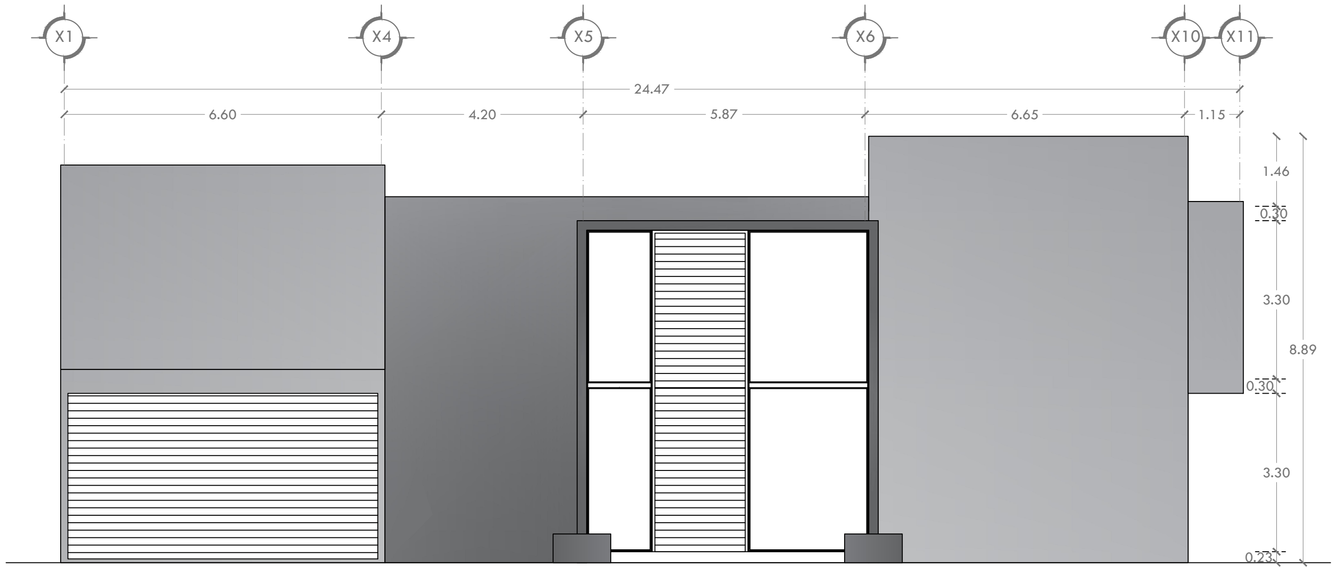
Vista-1 Proyecto CASA SELVA Nivel: 0 | Esc. S/E | Esc.G.
